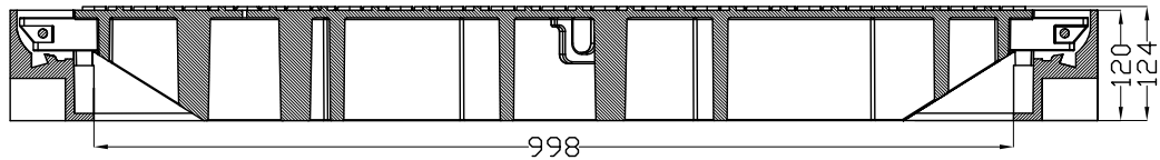
SEZIONE A-A
