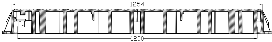
SEZIONE A-A
