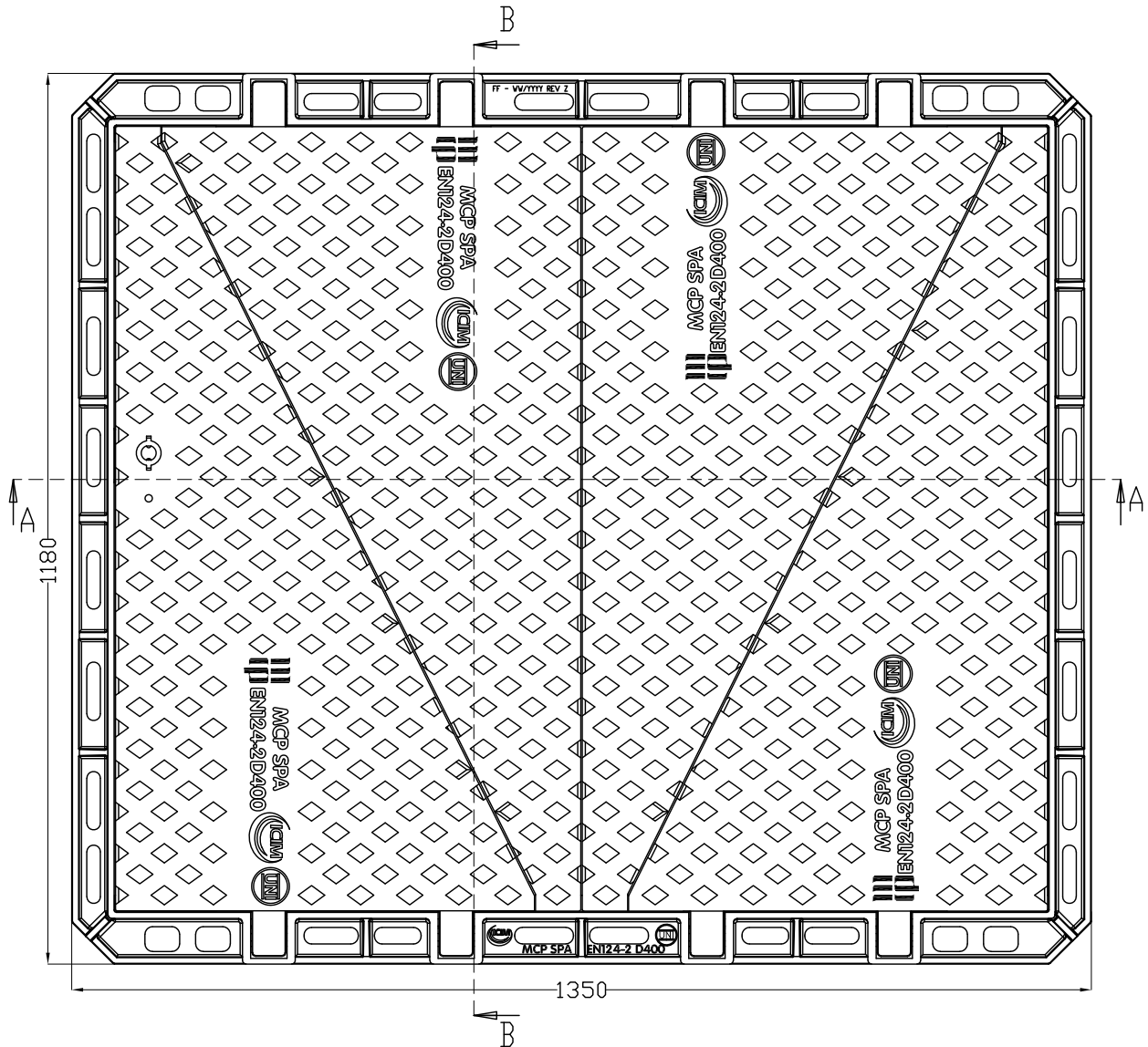
VISTA SUPERIORE
