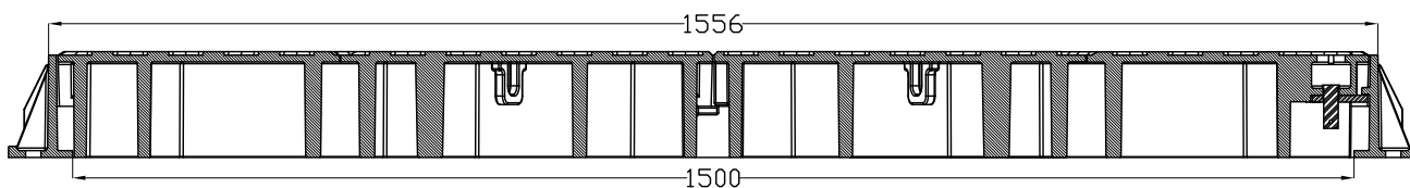
SEZIONE A-A
