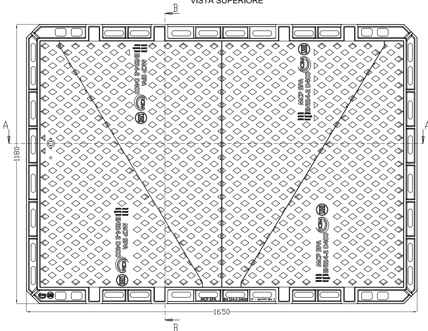
VISTA SUPERIORE
