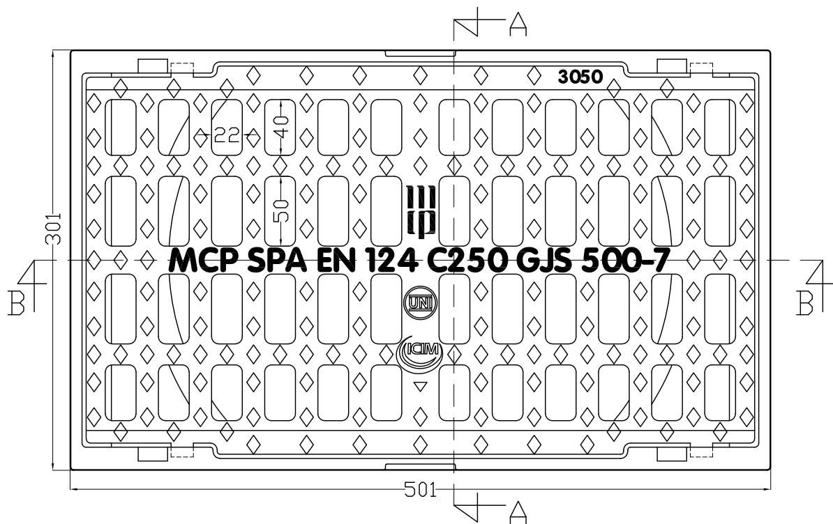
VISTA SUPERIORE
