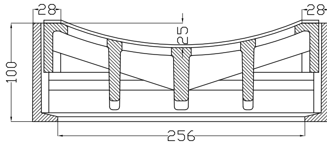
SEZIONE A-A
