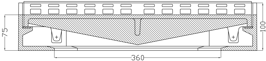
SEZIONE B-B
