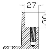
SEZIONE B-B
