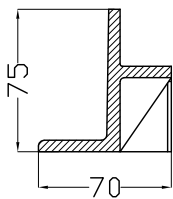
SEZIONE A-A
