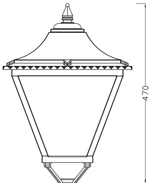
VISTA LATERALE
