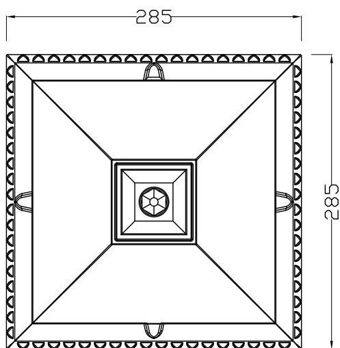
VISTA SUPERIORE
