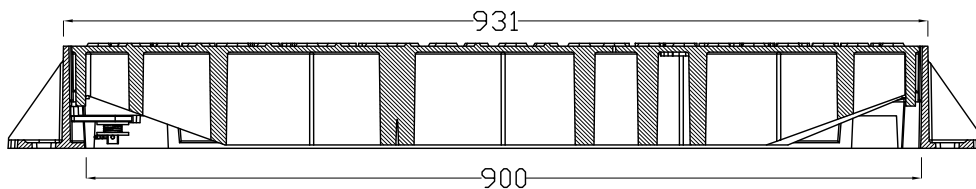
SEZIONE B-B
