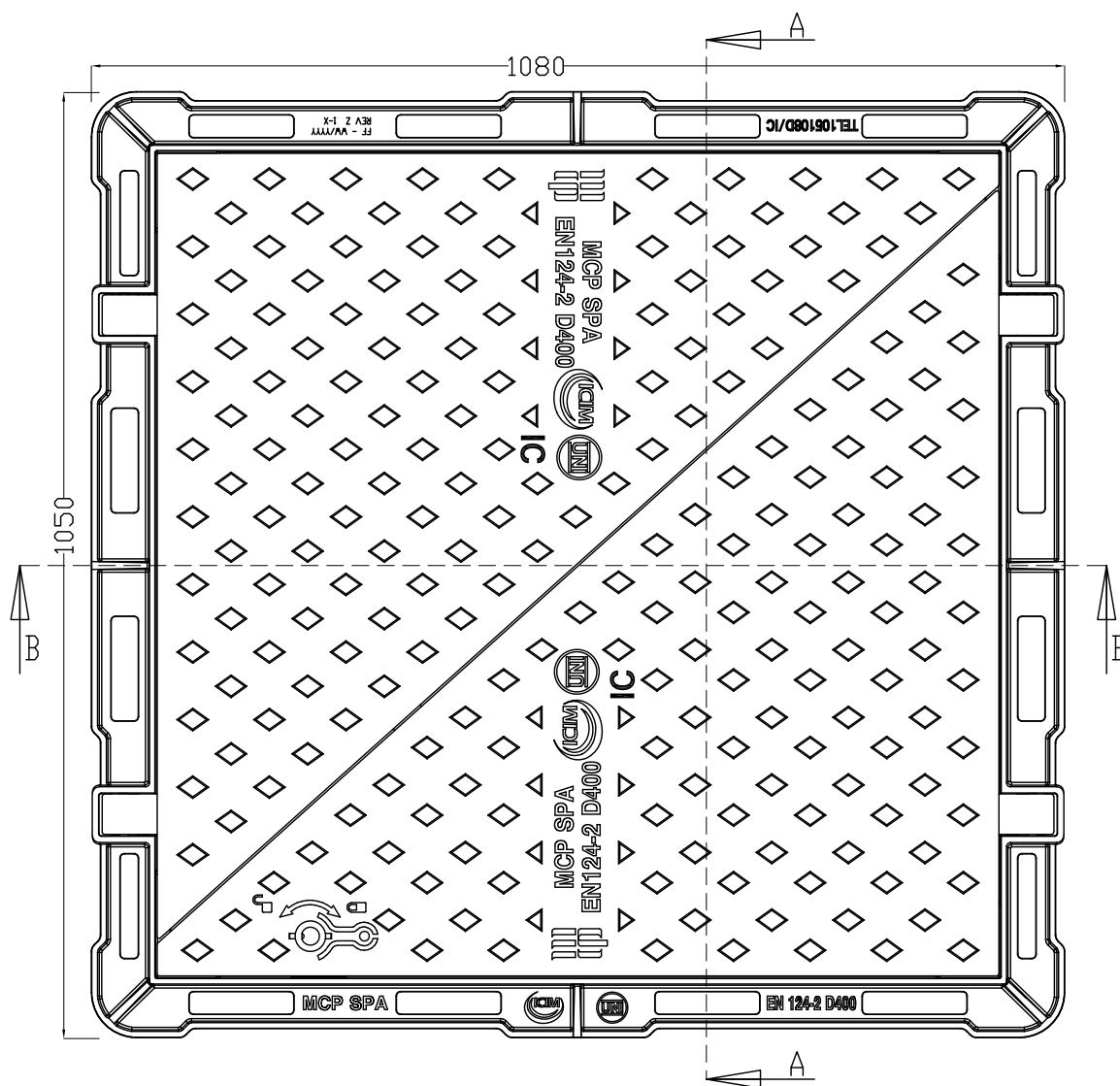
VISTA SUPERIORE
