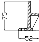
SEZIONE A-A
