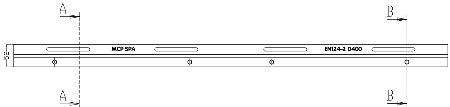
VISTA SUPERIORE
