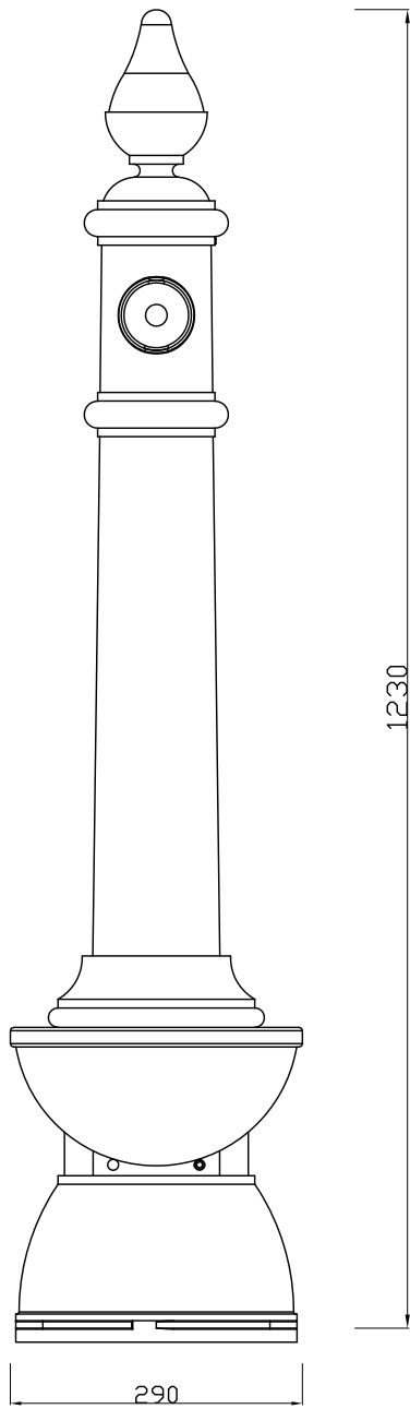
VISTA FRONTALE
