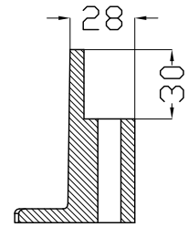
SEZIONE B-B
