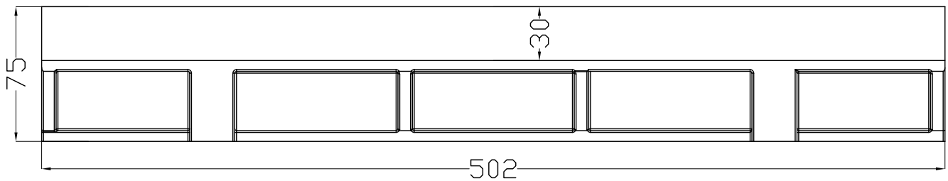
VISTA FRONTALE
