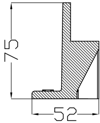
SEZIONE A-A
