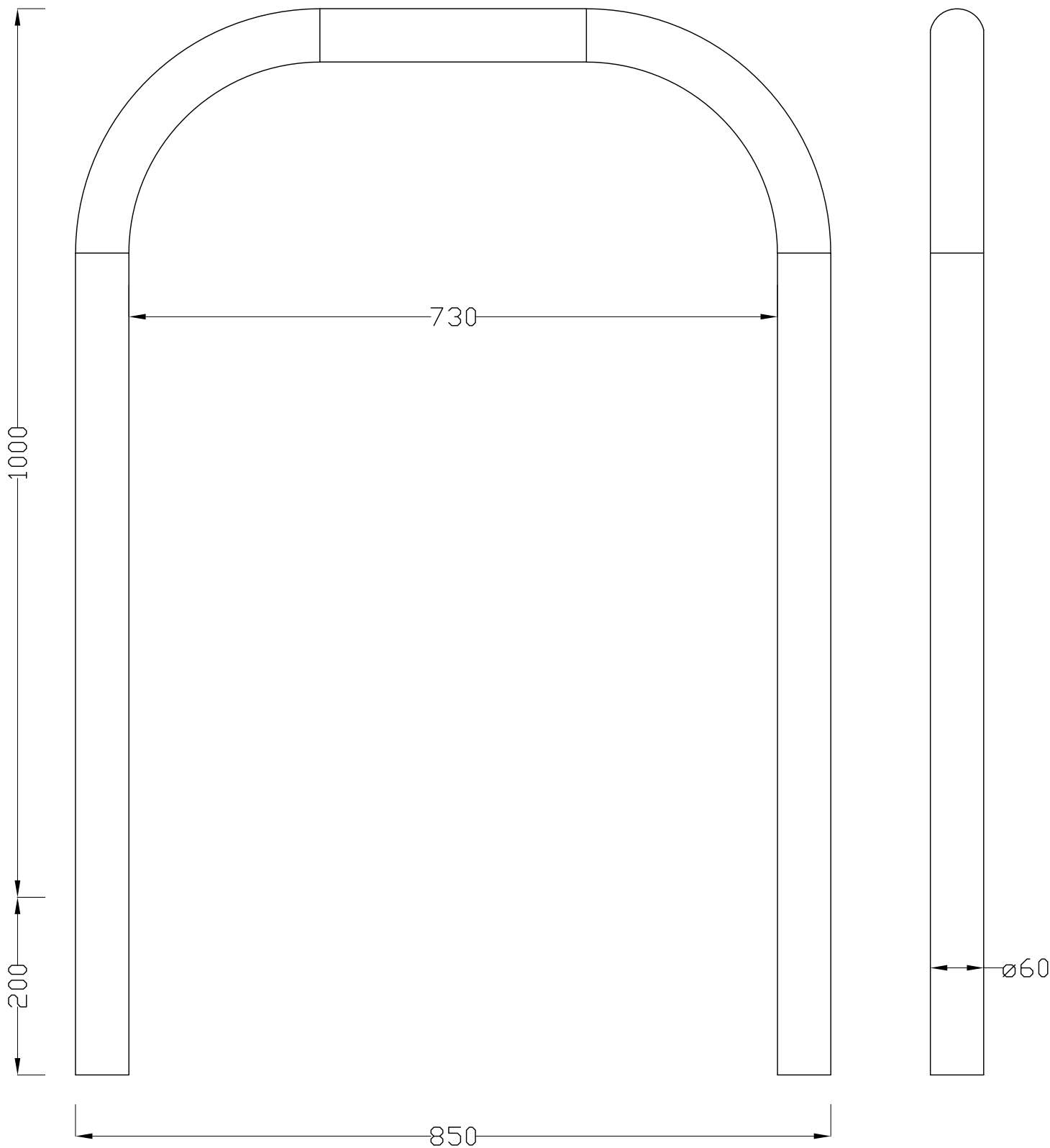
VISTA FRONTALE
